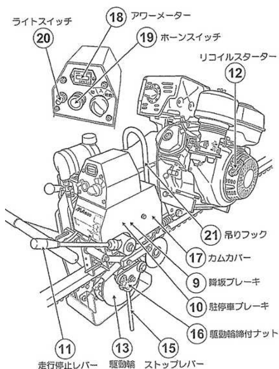
●イラストの牽引車はMA-600HSBを示しています。
