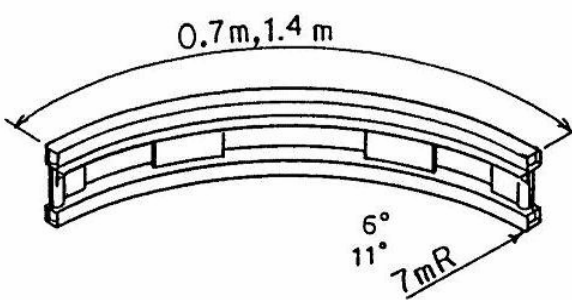
③内曲りレール (0.7m, 1.4m)
